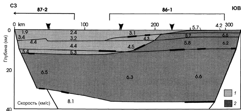
Рис. 9. Скоростная модель земной коры южной части Канадского бассейна по сейсмическому профилю 87-F [56]
