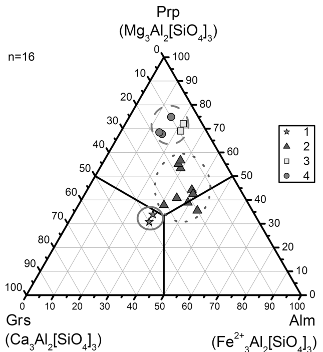
Рис. 4. Тройная диаграмма минерального состава гранатов из верхнемантийных ксенолитов. Миналы рассчитаны по [32]. На диаграмму нанесены только составы центральных частей гранатов
