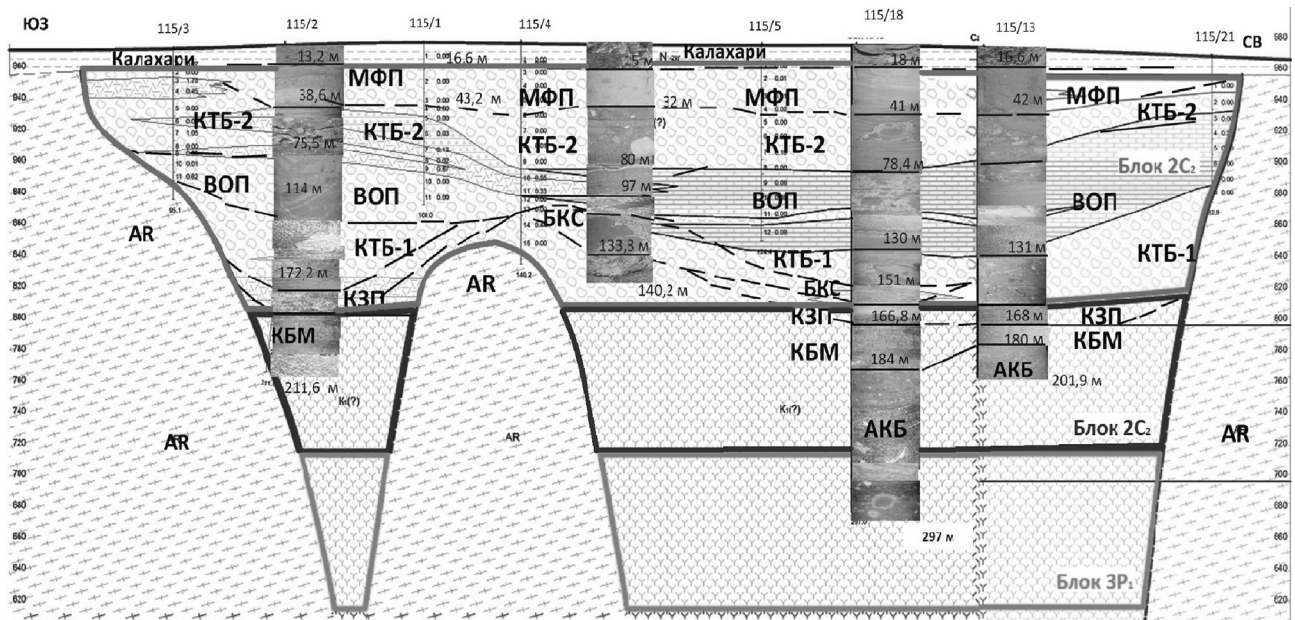
Рис. 3. Геологический разрез кимберлитовой трубки Кат-115 до глубины 350 м [4, с изменениями] Усл. обозн. см. на рис. 2
