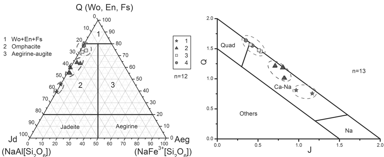
Рис. 7. Положение фигуративных точек клинопироксенов из ксенолитов эцлогитов и гранатовых лерцолитов на классификационных диаграммах [36]). На диаграмму нанесены составы только центральных частей клинопироксенов Усл. обозн. см. на рис. 4
