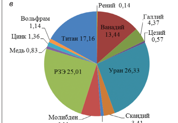
Рис. 3. Структура потенциальной стоимости запасов ДС (без учета Rb), % а – на всей поисковой площади, б – на участке 1, в – на участке 2
