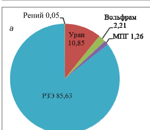
Рис. 1. Структура потенциальной стоимости запасов ДС, % а – на всей поисковой площади, б – на участке 1, в – на участке 2
