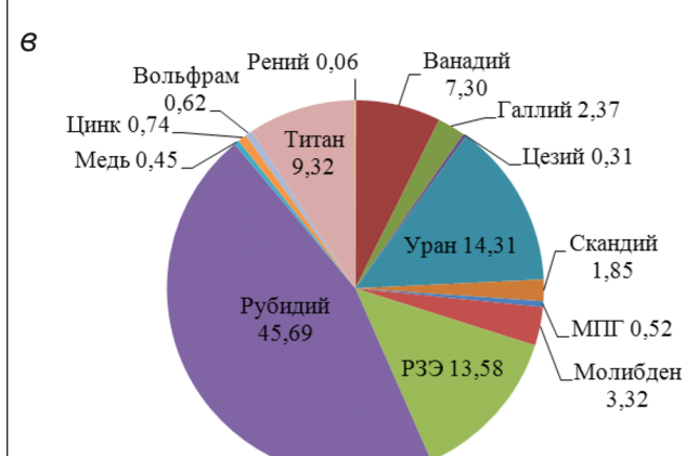
Рис. 1. Структура потенциальной стоимости запасов ДС, % а – на всей поисковой площади, б – на участке 1, в – на участке 2
