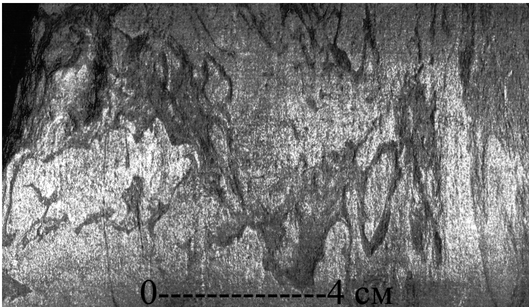
Рис. 6. Вихреподобные потоки туффзитов в песчанике. Темный цвет слоев обусловлен присутствием пылевидного графита. Яблоновский участок, пришлифовка образца из скв. 7, глубина 165 м (по К. Э. Якобсону и др. [19])
