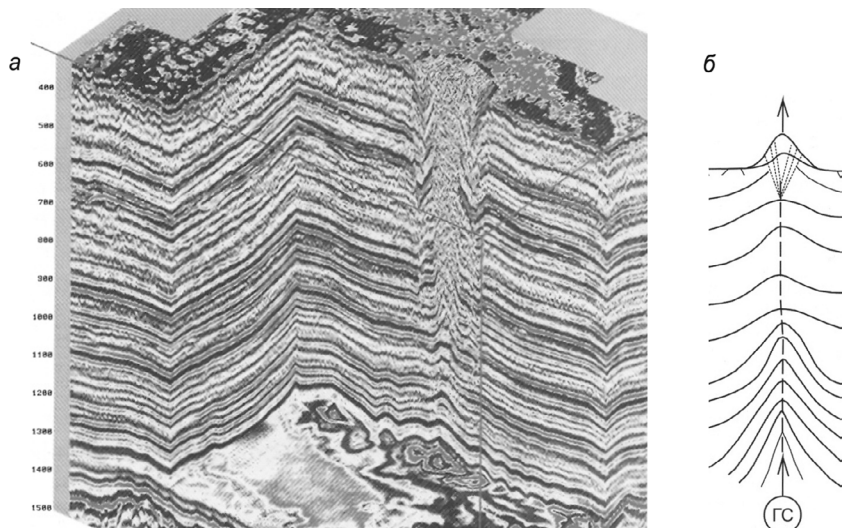
Рис. 8. Композиция горизонтального и вертикального сечения волнового поля по материалам 3D сейсморазведки, проходящего через геосолитонную трубку. Пульгынская площадь – a , теоретическая модель салитона – б (по В. М. Мерера [9])
