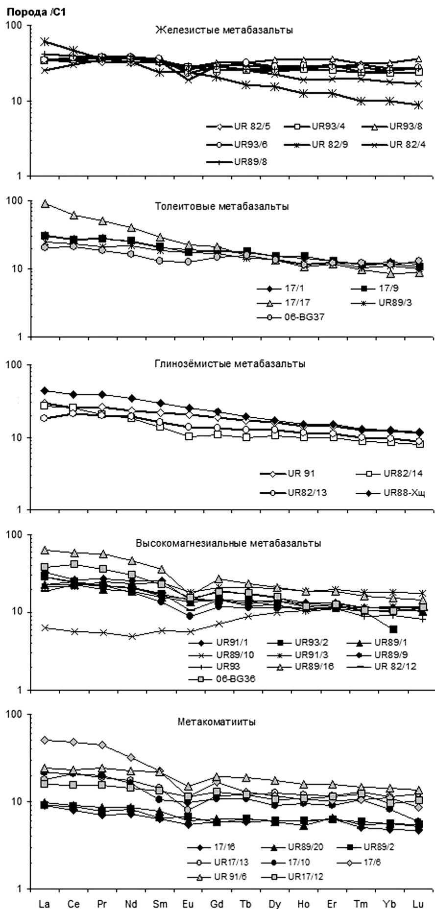
Рис. 4. Распределение РЗЭ в петрохимических группах кристаллосланцев (06-BG36 из работы [15])
