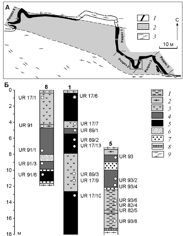
Рис. 2. Геологическое строение северной части карьера Одесский днестровско-бугской серии (А) и деталиные разрезы, показывающие объемы кристаллосланцев различного состава, их перемежаемость друг с другом и с метаморфизованными осадочными породами (Б)
