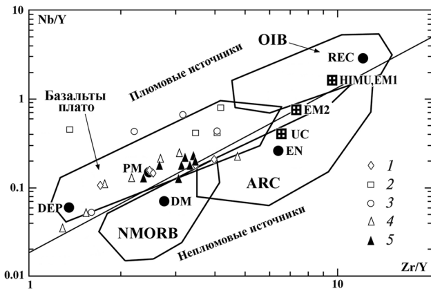
Рис. 7. Положение кристаллоандезитов днестровско-бугской серии на диаграмме Nb/Y–Zr/Y [17]. Точки метабазальтов и метакоматиитов располагаются в поле (или вблизи него) базальтов плато – производных глубинного источника (DEP) 1–4 – метабазальты (1 – железистые, 2 – толеитовые, 3 – глинозёмистые, 4 – высокомагнезиальные); 5 – метакоматииты
