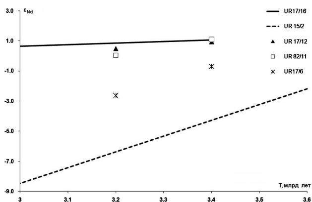
Рис. 5. Диаграмма \epsilon_{\text{Nd}}-T для коматиитов и гнейсэндербита, показывающая принципиальную возможность нарушения Nd изотопной системы коматиитов за счет различной степени ассимиляции коматиитом (UR 17/16) древнего гнейсэндербита (UR 15/2)
