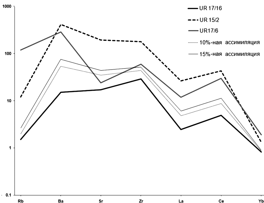
Рис. 6. Расчет баланса элементов при двухкомпонентном смешении гнейсэндербита (UR 15/2) и коматиита (UR 17/16)
