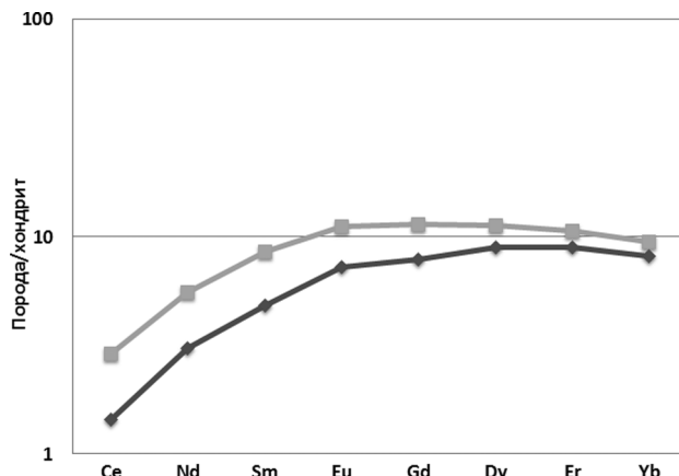
Рис. 3. Третичные, или мезозойские, «коматииты» острова Горгона [15]
