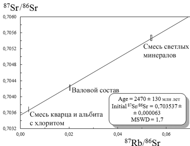
Рис. 3. Изотопная Rb-Sr изохрона для образца пропилита V1111
