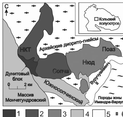
Рис. 1. Расположение Мончеплутона и массива Вуручуайвенч в нем [7]
