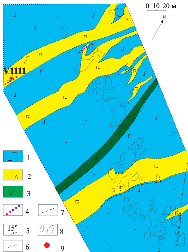
Рис. 2. Схема участка детального изучения в юго-западной части массива Вуручайвенч [7]
