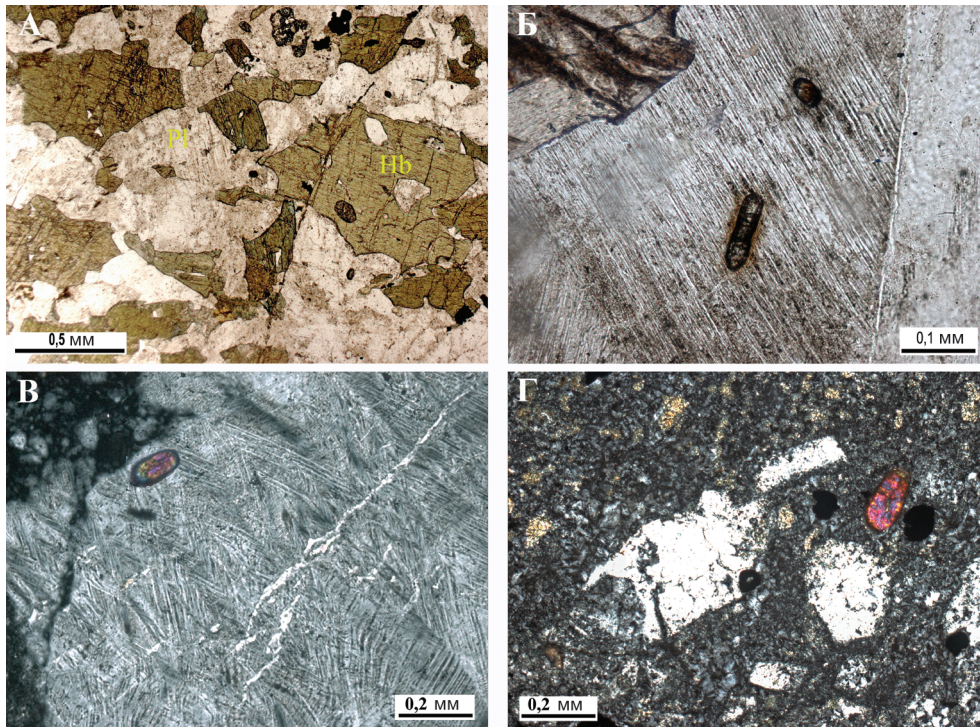
Рис. 3. Циркон в ударно-метаморфизованных породах разреза ВГС (микрофотографии шлифов; А, Б – без анализатора, В, Г – николи Х)
