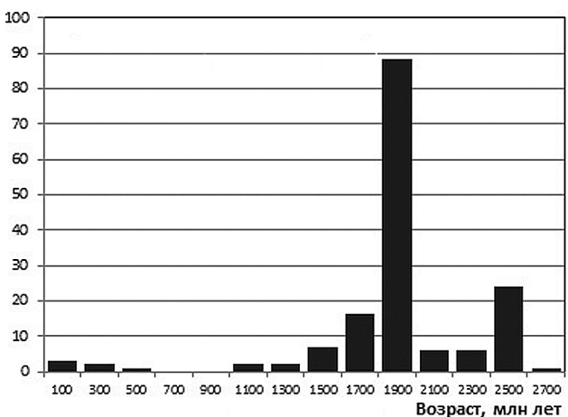
Рис. 7. Гистограмма ^{207}Pb/^{206}Pb возрастов (древнее 1,0 млрд лет) и точек нижних пересечений дискордий (менее 1,0 млрд лет) проанализированных цирконов
