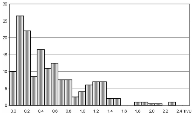
Рис. 6. Гистограмма значений Th/U отношения в цирконах из пород кристаллического фундамента Воротиловского выступа
