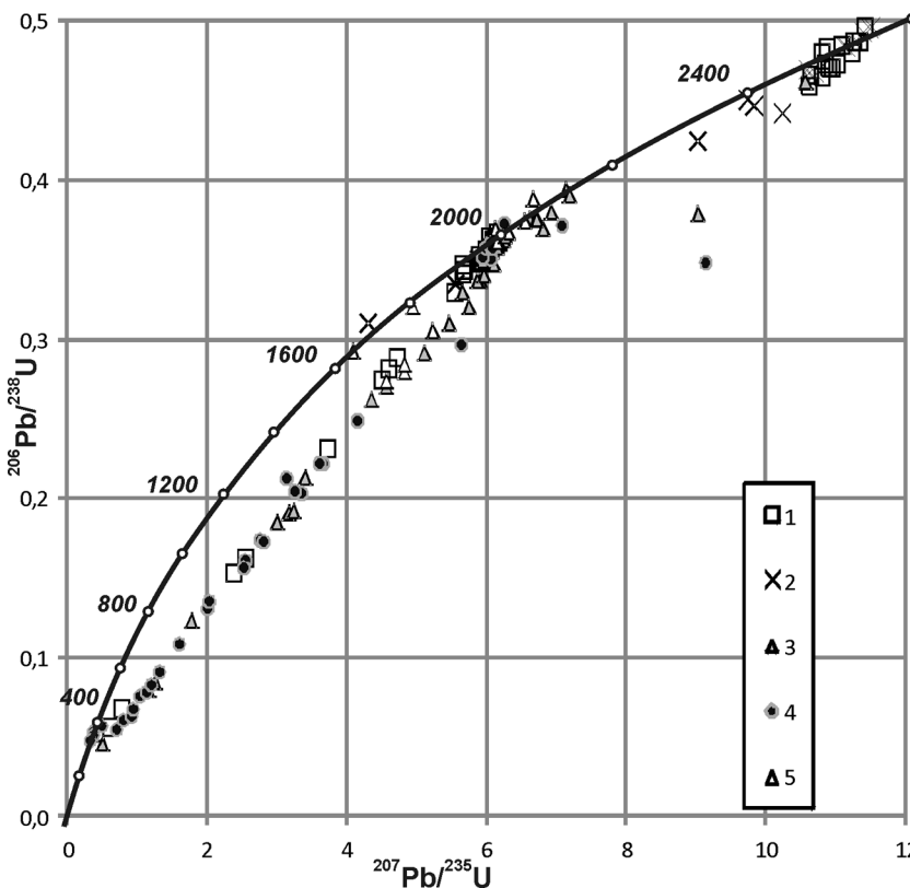
Рис. 9. Сводная ^{206}\text{Pb}/^{238}\text{U} – ^{207}\text{Pb}/^{235}\text{U} диаграмма для всех исследованных цирконов из пород Воротиловского выступа 1 – слабо ударно-метаморфизованные плагиогнейсы и амфиболиты с глубин ниже 5300 м; 2 – долериты; 3 – умеренно ударно-метаморфизованные гнейсы и граниты с глубин 3000–5250 м; 4 – интенсивно ударно-метаморфизованные гнейсы из прикровлевой части аутигенной брекчии и 5 – зювита
