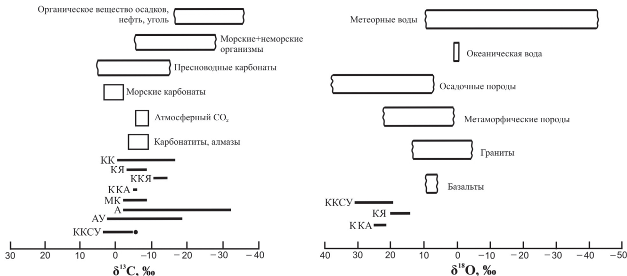
Рис. 4. Вариации \delta^{13}\text{C} и \delta^{18}\text{O} для карбонатов из разных источников и пород района горы Благодать. График Й. Хевса (2009) с дополнениями
