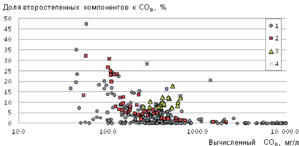
Рис. 2. Доля микрокомпонентов по отношению к CO_B
