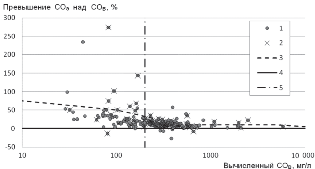
Рис. 1. Разность между CO_3 и CO_B по отношению к CO_B
