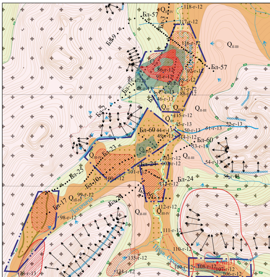
Рис. 4. Прогнозная схема рудопоявления урана Орогочинское
