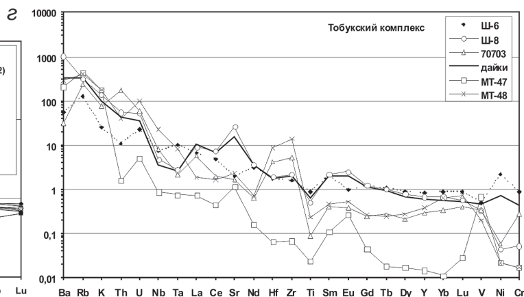
Рис. 5. Петрогеохимическая характеристика горных пород мезозойских комплексов Алдана
