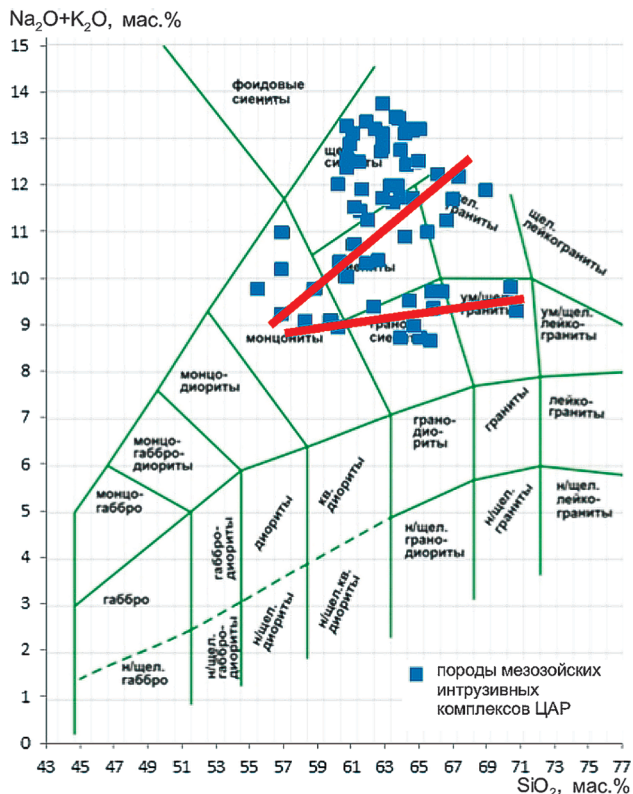
Рис. 4. Положение фигуративных точек состава исследуемых мезозойских интрузивных пород ЦАР на диаграмме TAS. Красными линиями обозначены тренды изменения составов пород
