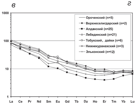
Рис. 5. Петрогеохимическая характеристика горных пород мезозойских комплексов Алдана
