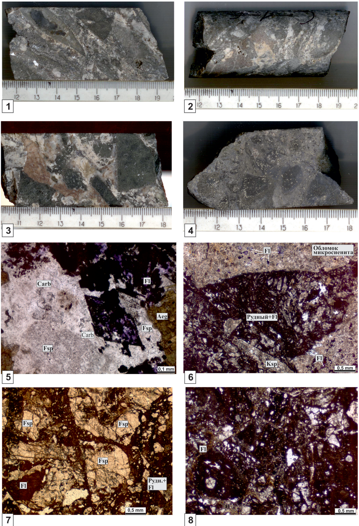
Рис. 5. Гидротермальные брекчии – фотографии
