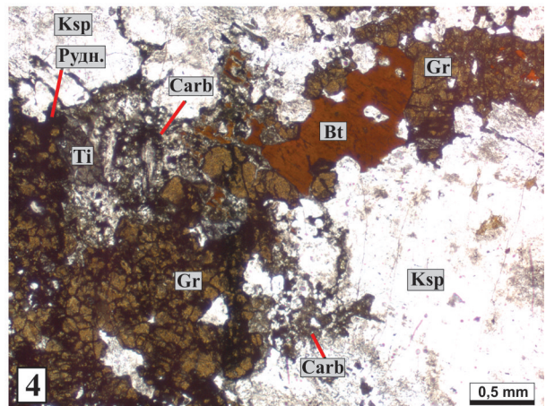
Рис. 4. Гранатовые брекчии (образцы С-1-79 м и С-1-234 м и шлифы к ним) – фотографии
