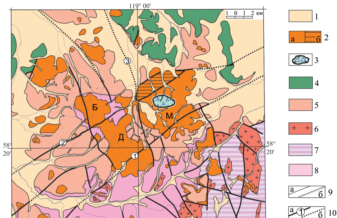
Рис. 1. Схематическая геологическая карта Мурунского магматического узла (по данным Л.Б. Маркарева и др., 2013)
