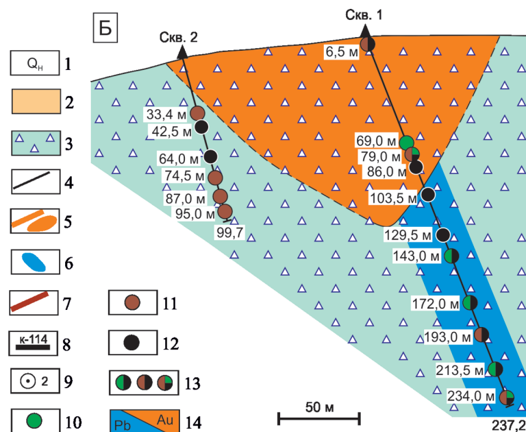
Рис. 2. Схематическая геологическая карта Маломурунской брекчиевой трубки с данными по рудоносности (А) и разрез по скважинам (Б), по материалам П.В. Ломыга, 2013, с дополнениями авторов
