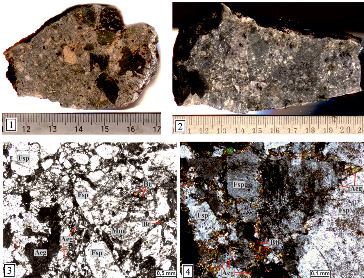
Рис. 3. Эгириновые брекчии (образцы 1360 и 1453 и шлифы к ним) – фотографии
