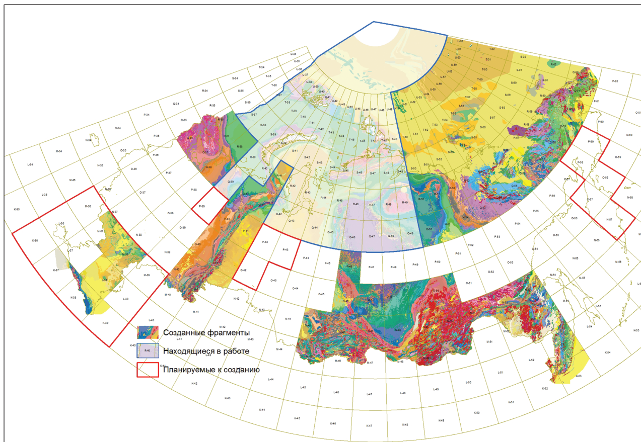
Рис. 7. Бесшовные геологические карты масштаба 1 : 1 000 000 территории Российской Федерации и ее континентального шельфа
