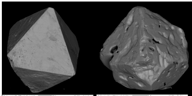
Рис. 1. Внешние формы кристаллов пироклора (обратно-рассеянные электроны). Пробы 1069/2 и 1066/3 из массива Ковдор (гора Воцу-Вара)
