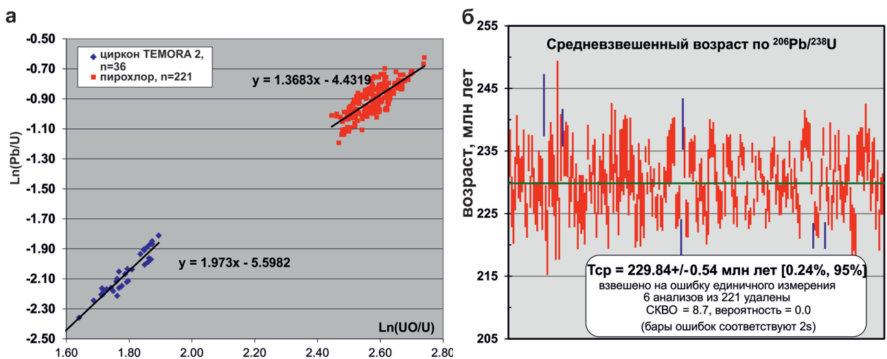
Рис. 4. Характеристика U-Pb изотопного анализа единичных зерен внутрилабораторного стандарта пирохлора-331 с помощью вторично-ионного масс-спектрометра SHRIMP II
