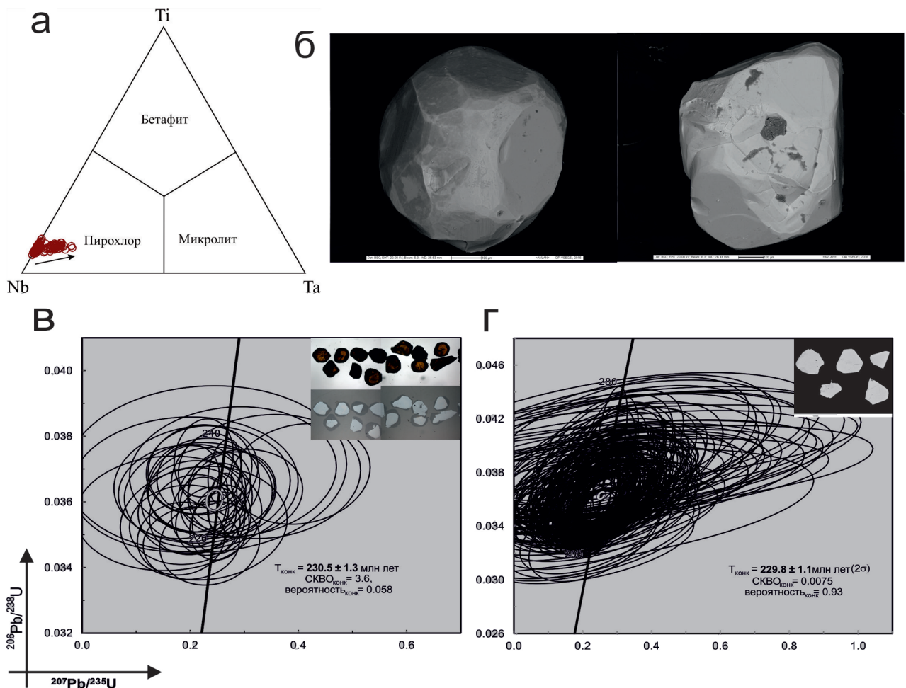
Рис. 3. Минералого-геохимическая характеристика внутрилабораторного стандарта пирохлора-331
