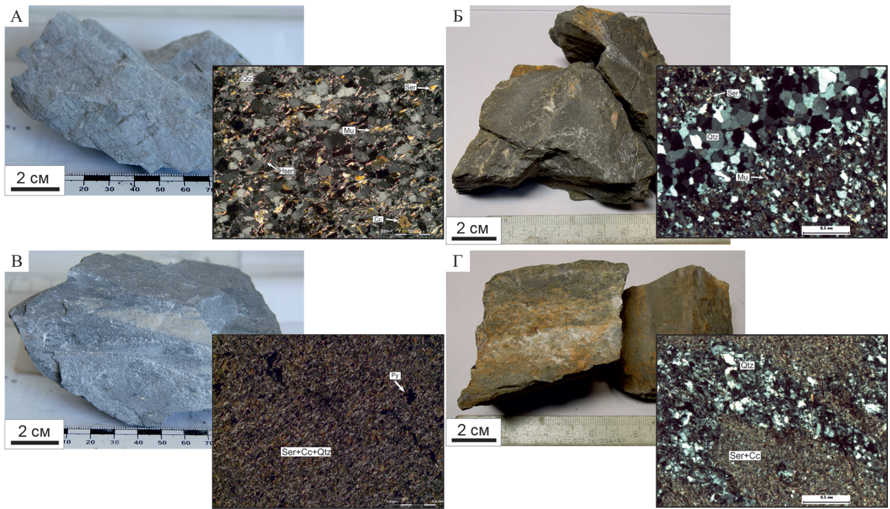
Рис. 2. Безуглеродистые березиты
