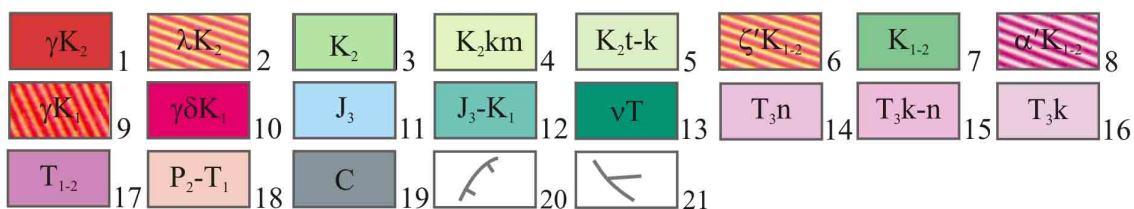
Рис. 1. Схема расположения Катумского потенциально урановородного района (по материалам ФГБУ «ВСЕГЕИ», ВИМС, ВИРГ, ФГУП «Дальгеофизика», масштаб 1 : 500 000
