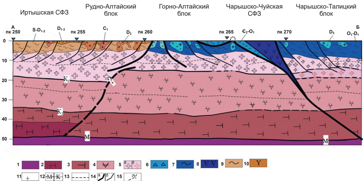
Рис. 5. Глубинный геолого-геофизический разрез Горно-Рудно-Алтайского блоков в сечении профиля ГСЗ-МОВЗ «Базальт»
