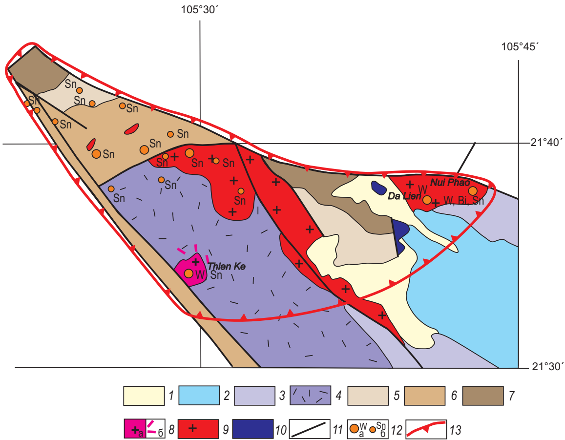
Рис. 4. Олово-вольфрамовый рудный узел Там Зао
