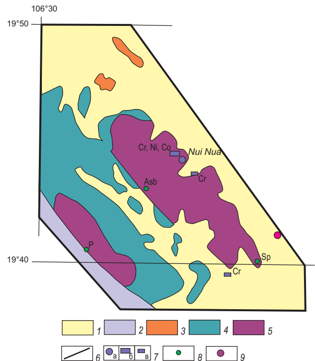
Рис. 6. Никель-хромовый рудный узел Нуи Нуа
