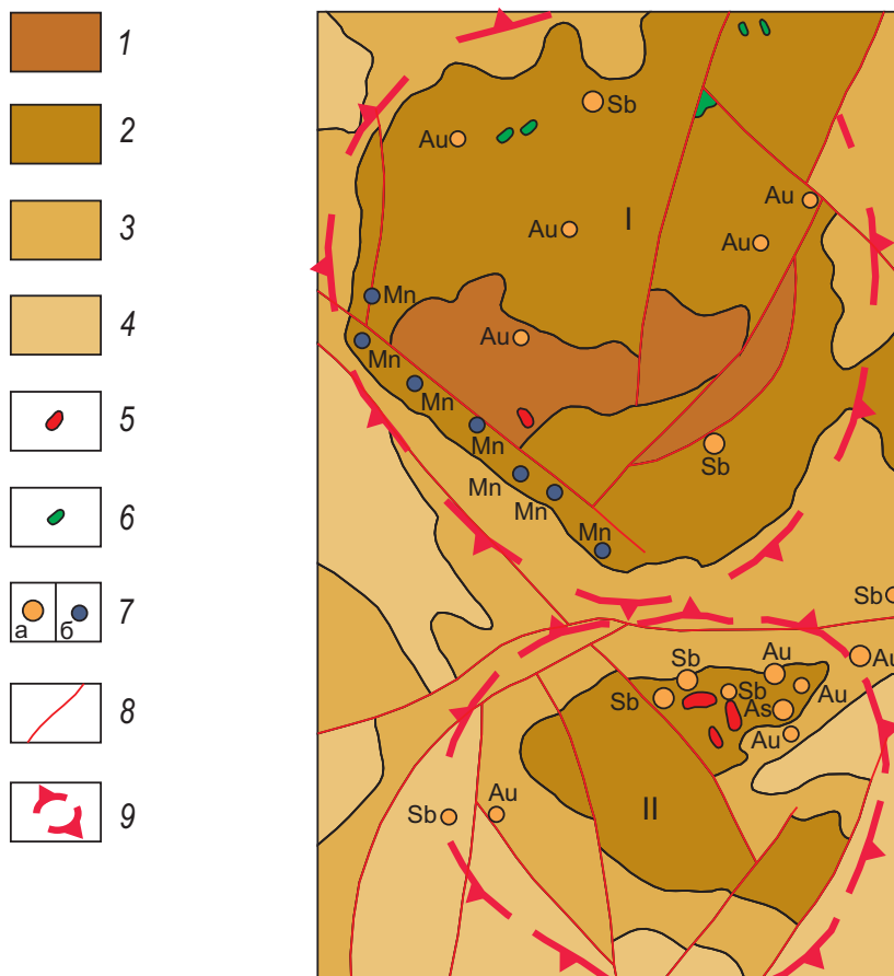
Рис. 2. Золото-сурьмяный рудный район Чием Хоа с рудными узлами Ланг Вай и Ланг Кан. Масштаб 1 : 200 000
