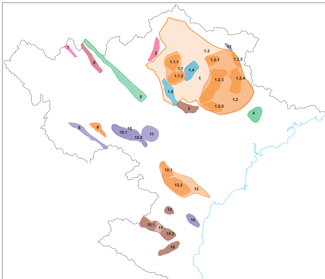
Рис. 1. Схема минерагенического районирования территории Тей Бак. Масштаб 1 : 2 000 000
