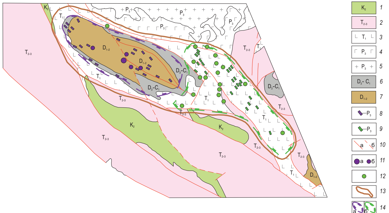
Рис. 5. Платинометалльно-медно-никелевый рудный район Бан Фук. Масштаб 1 : 200 000
