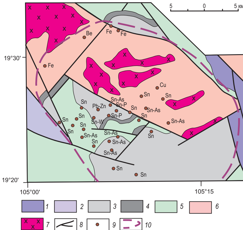
Рис. 3. Потенциально оловорудный узел Куи Хоп
